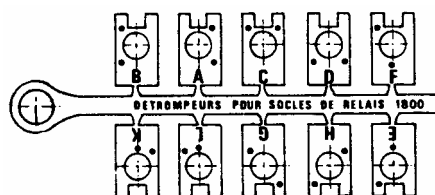
plaquette de détrompage 9871 disponible en couleur BLEU (instantané), VERT (bistable), MARRON (temporisé) ou ROUGE (bas niveau)
