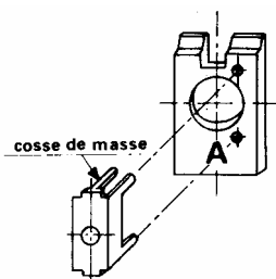
détrompeur sur relais
