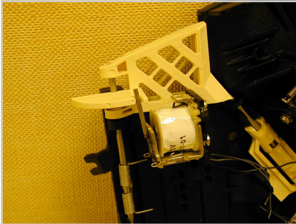
Solenoid used : 7613
